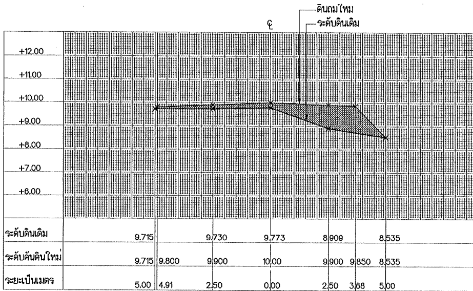
รูปตัด STA. 0+150
