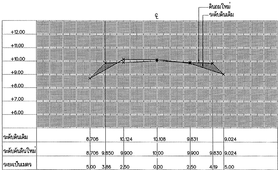
รูปตัด STA. 0+700
