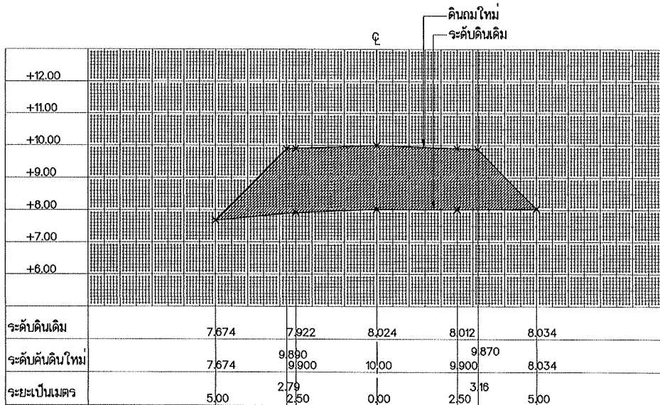
รูปตัด STA. 1+075
