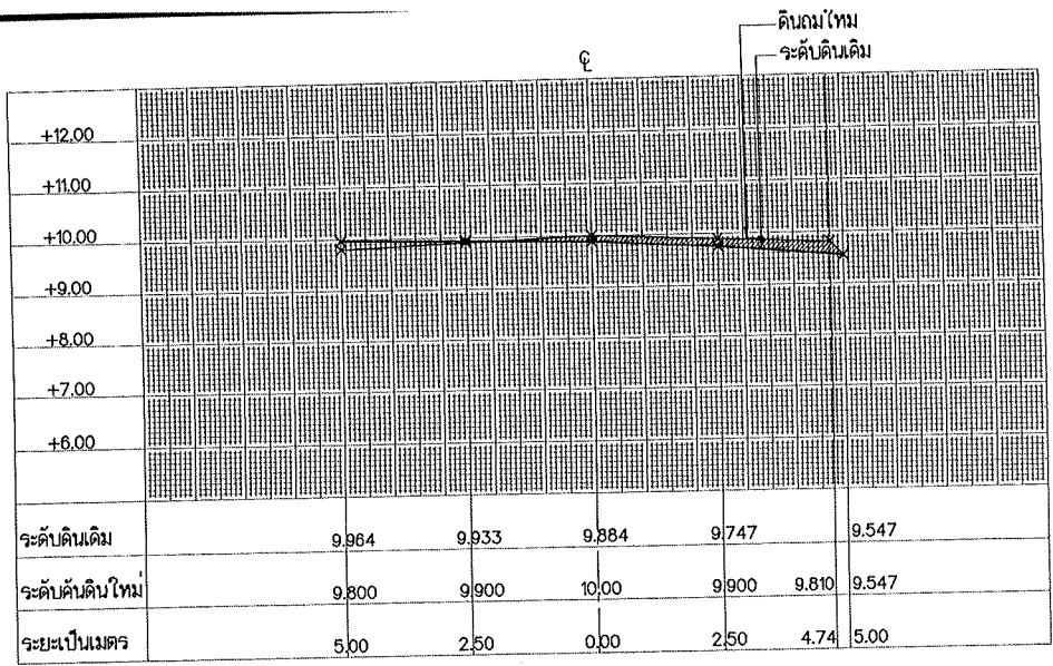
รูปตัด STA. 0+375
