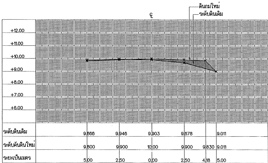
รูปตัด STA. 0+625
