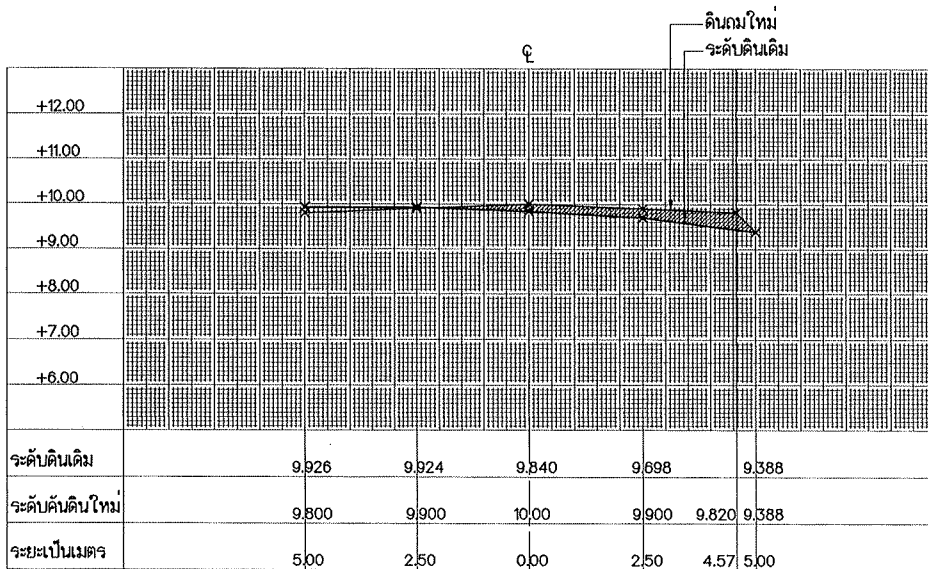
รูปตัด STA. 0+550
