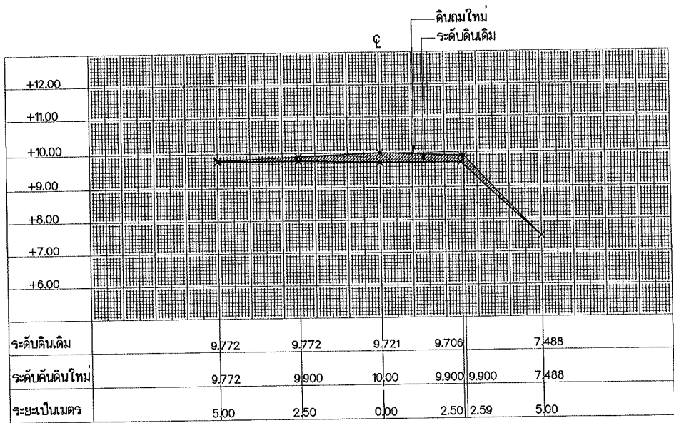
รูปตัด STA. 0+425
