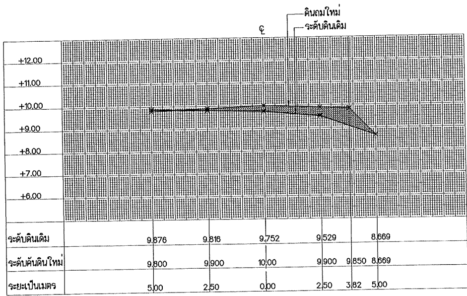
รูปตัด STA. 0+400
