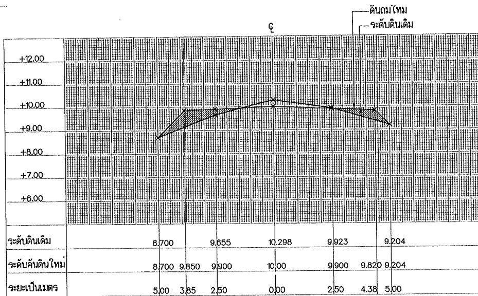
รูปตัด STA. 0+075
