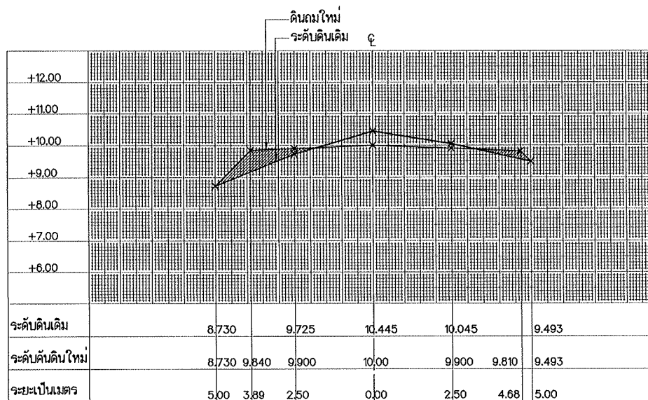
รูปตัด STA. 0+025
