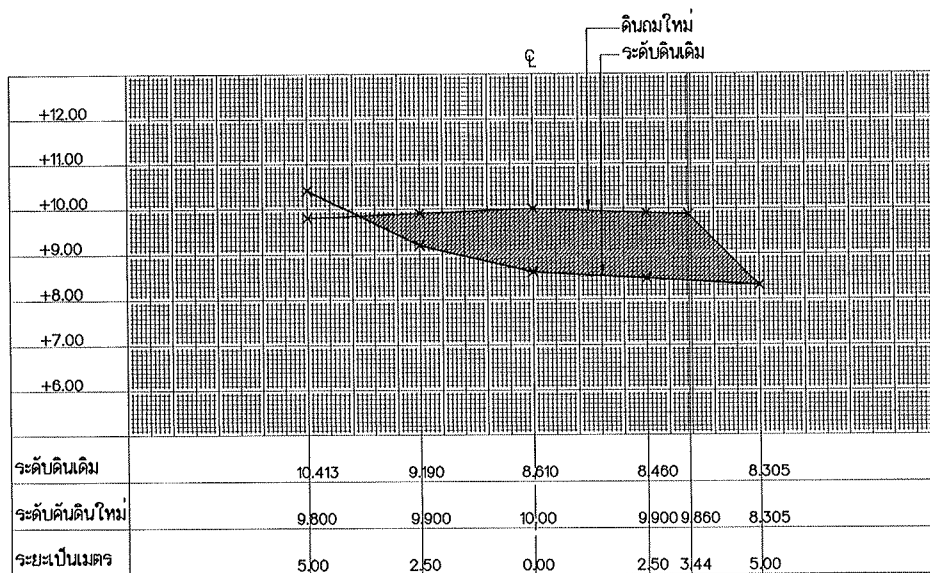
รูปตัด STA. 0+100
