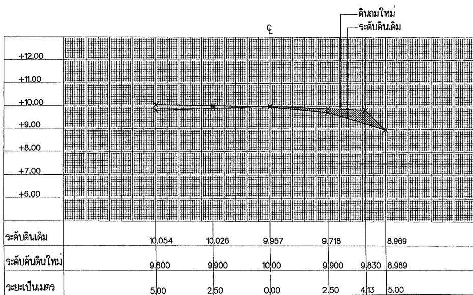
รูปตัด STA. 0+350
