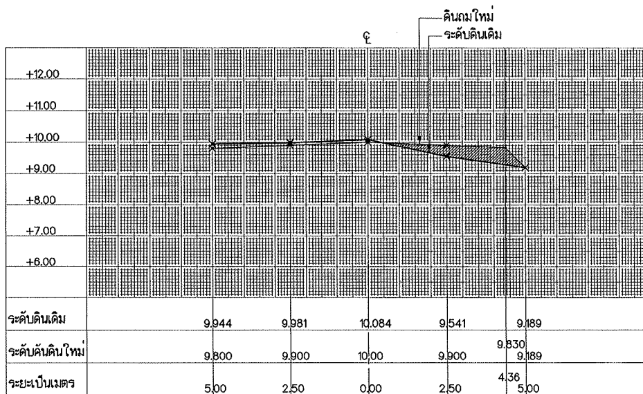
รูปตัด STA. 0+800
