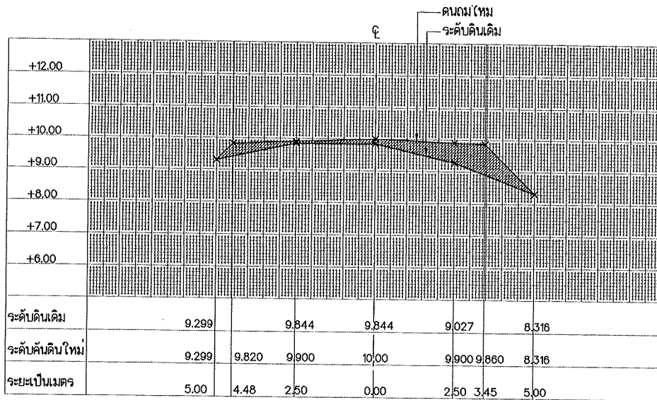
รูปตัด STA. 0+225
