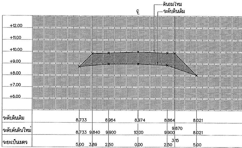
รูปตัด STA. 0+900
