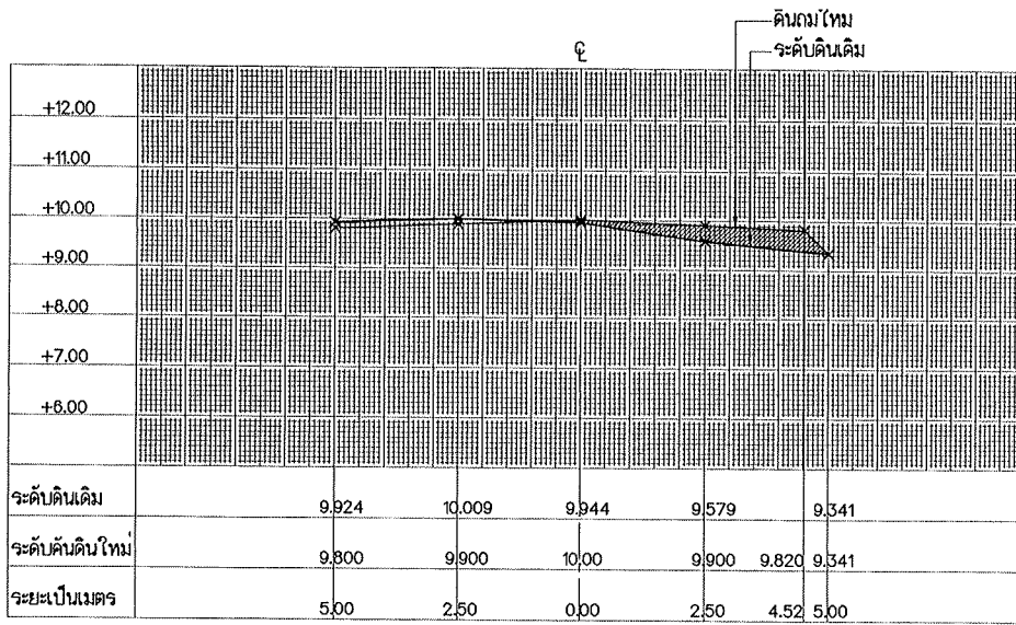
รูปตัด STA. 0+300
