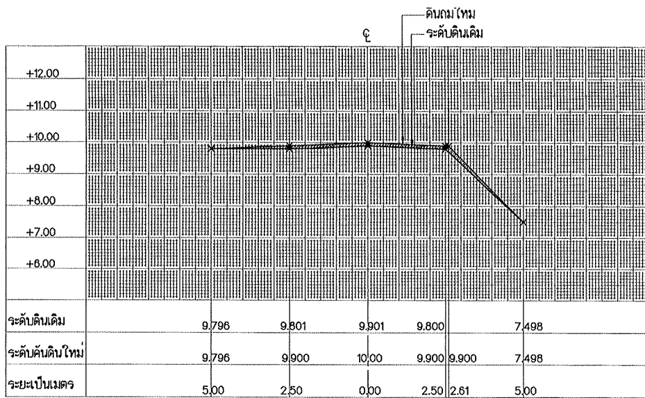
รูปตัด STA. 0+450
