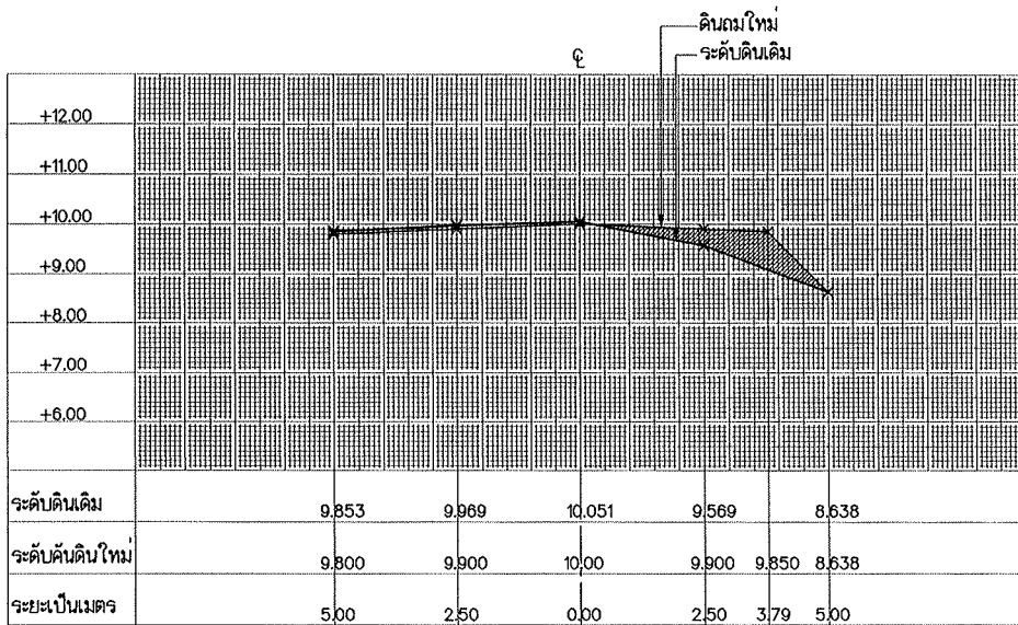
รูปตัด STA. 0+775
