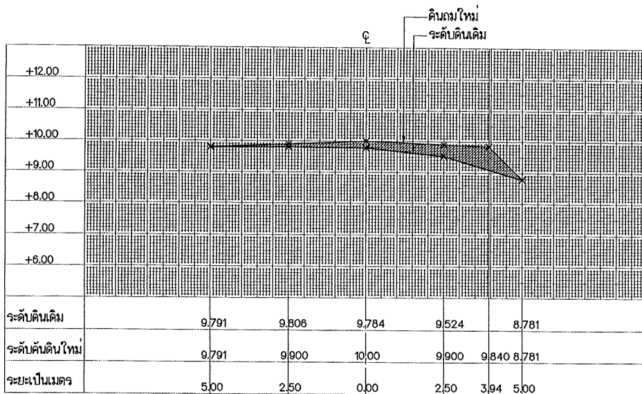
รูปตัด STA. 0+250
