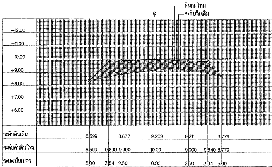
รูปตัด STA. 0+975
