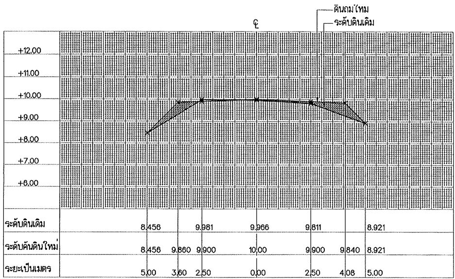
รูปตัด STA. 0+675
