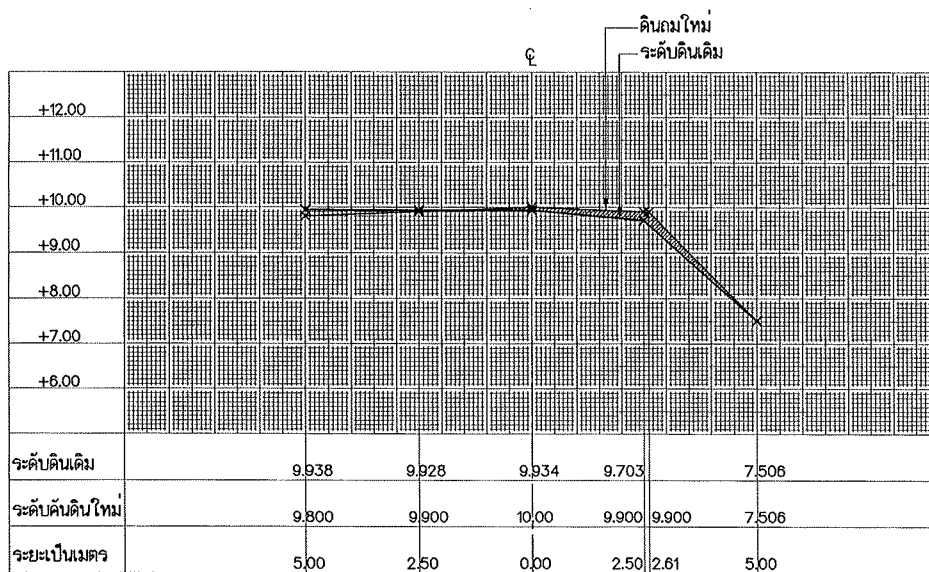
รูปตัด STA. 0+500
