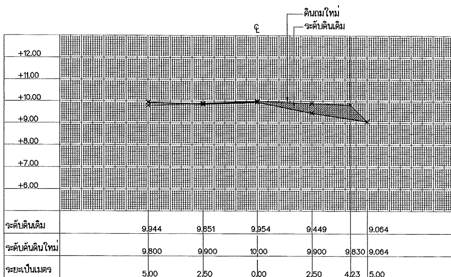
รูปตัด STA. 0+275
