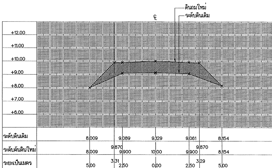
รูปตัด STA. 1+025
