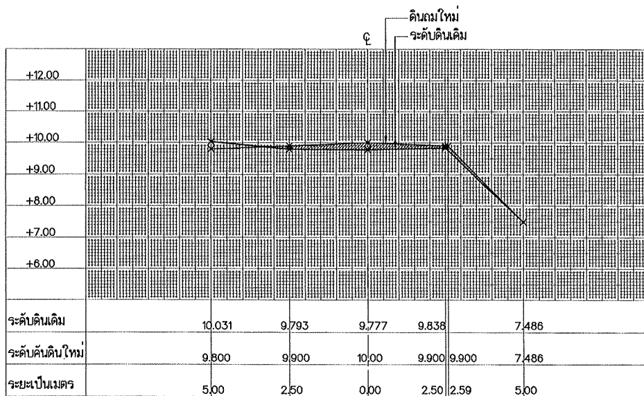
รูปตัด STA. 0+475
