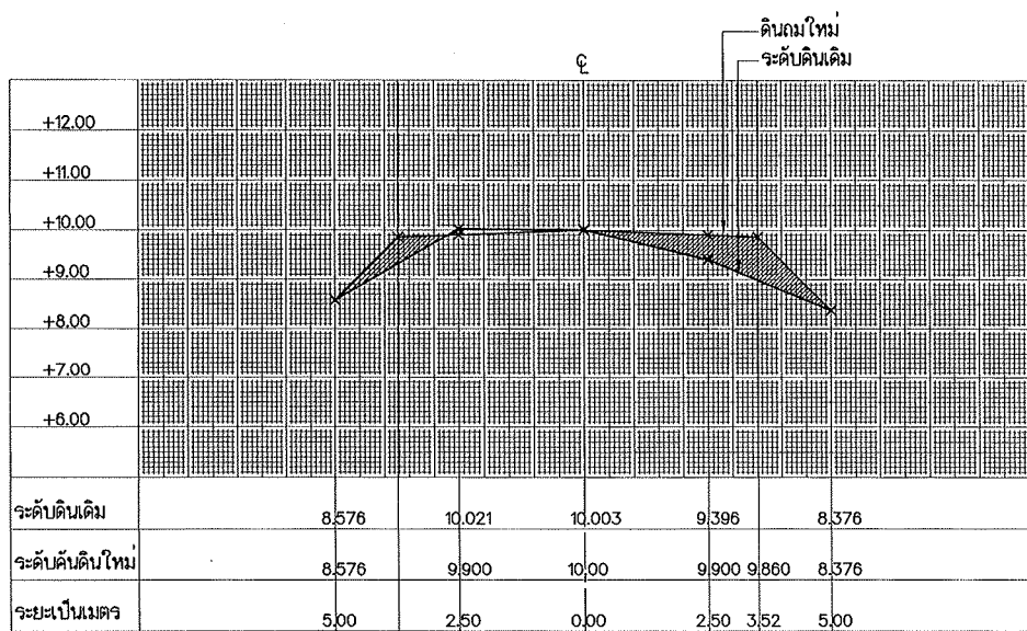
รูปตัด STA. 0+650
