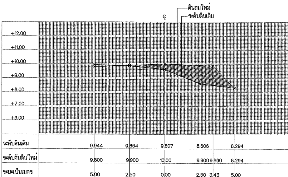
รูปตัด STA. 0+175
