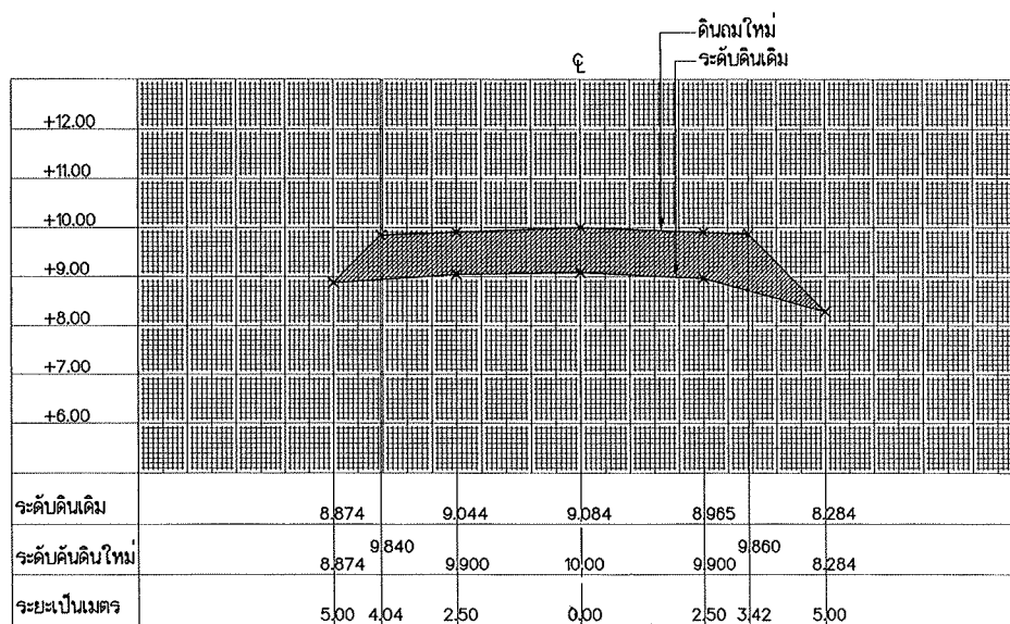
รูปตัด STA. 0+875
