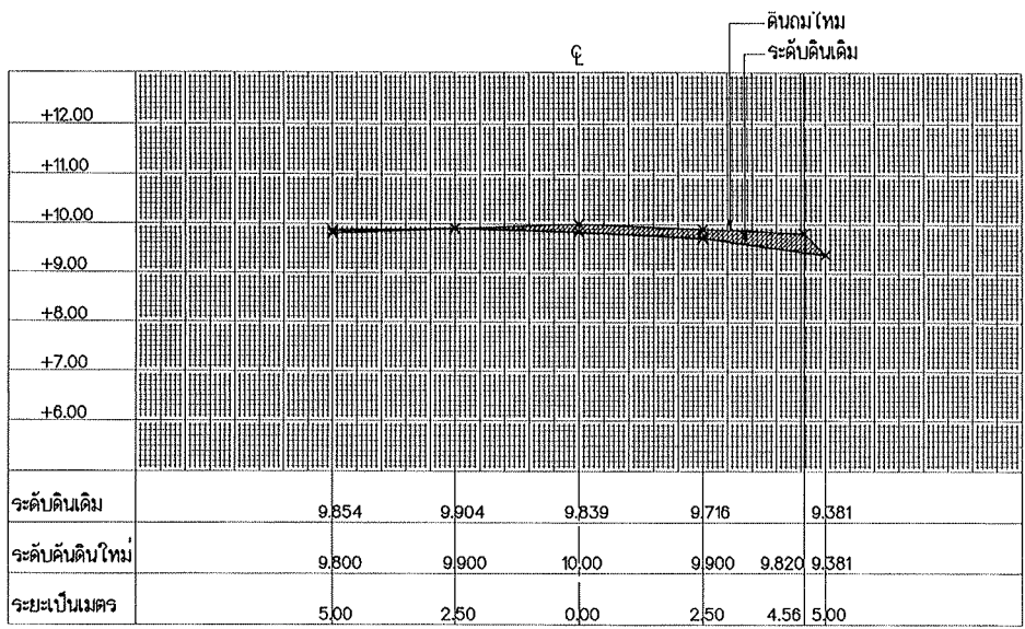
รูปตัด STA. 0+600
