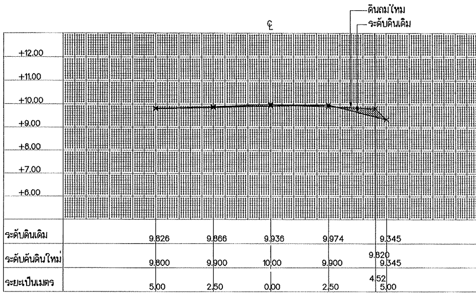
รูปตัด STA. 0+750
