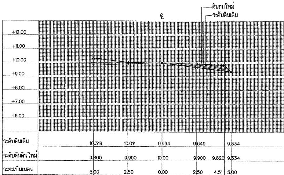
รูปตัด STA. 0+325
