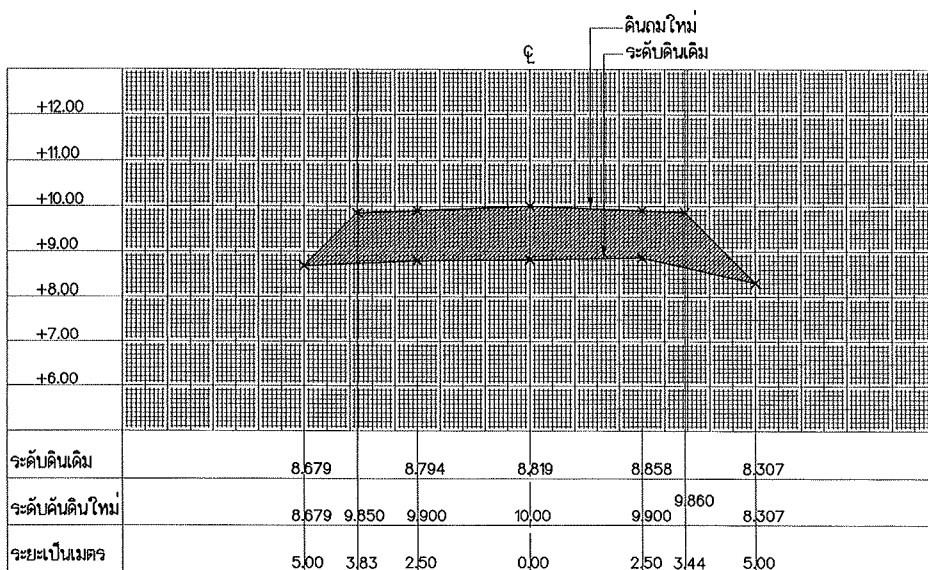
รูปตัด STA. 0+950
