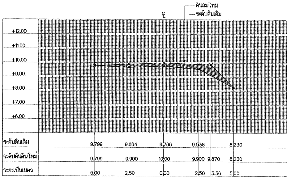
รูปตัด STA. 0+525
