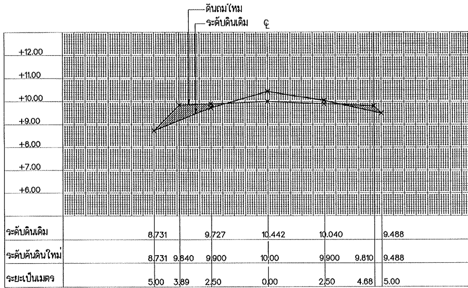
รูปตัด STA. 0+000
