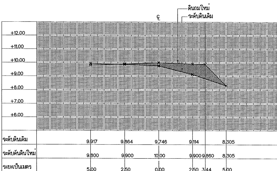
รูปตัด STA. 0+200
