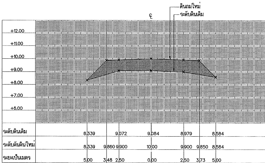
รูปตัด STA. 1+000
