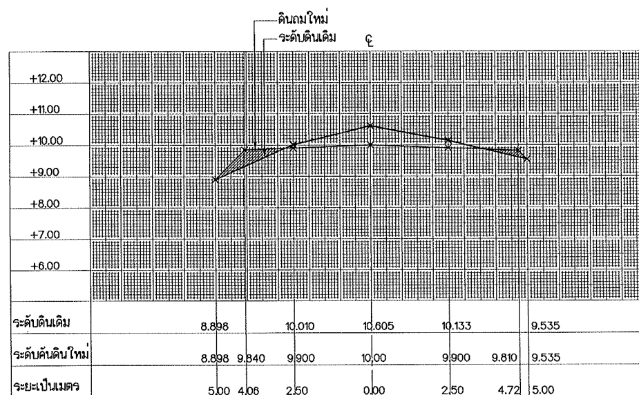
รูปตัด STA. 0+050
