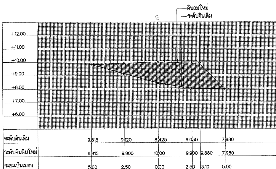
รูปตัด STA. 0+125
