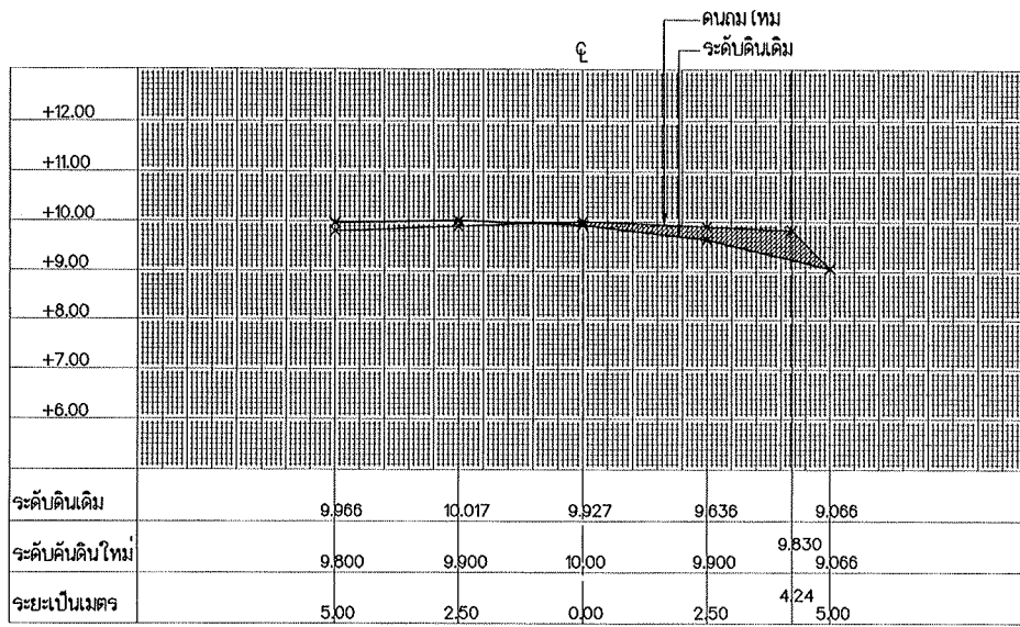
รูปตัด STA. 0+825
