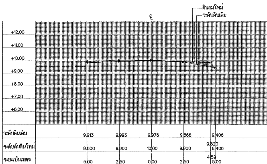
รูปตัด STA. 0+725
