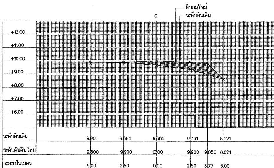
รูปตัด STA. 0+575
