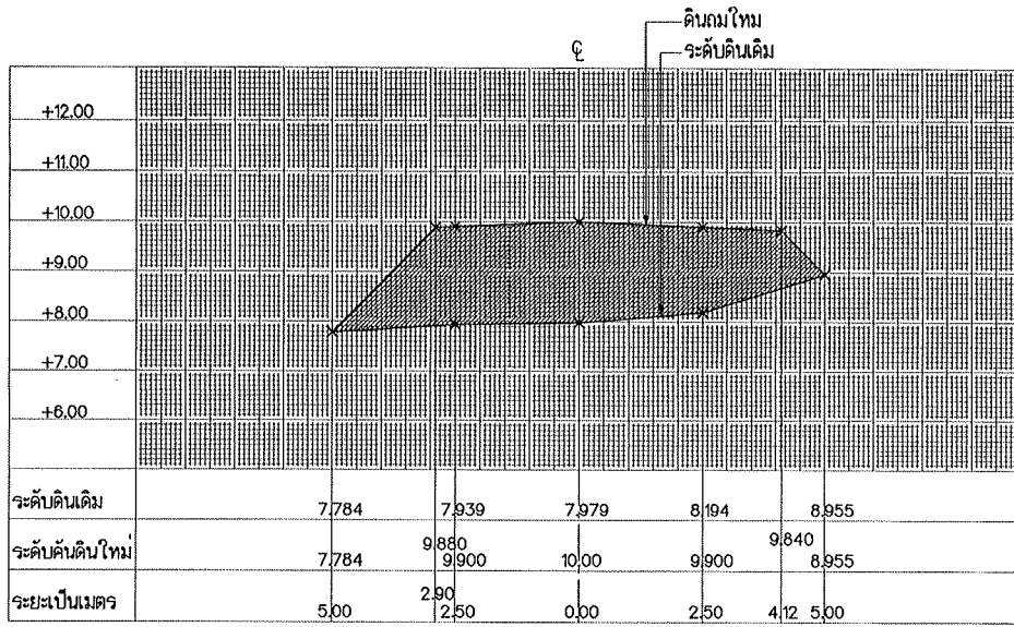
รูปตัด STA. 1+050
