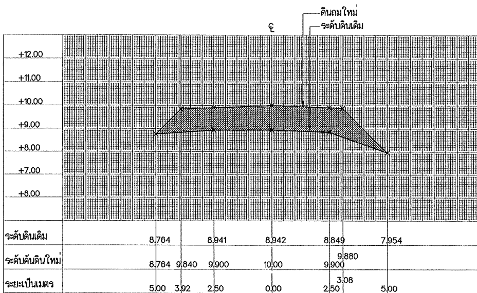
รูปตัด STA. 0+925
