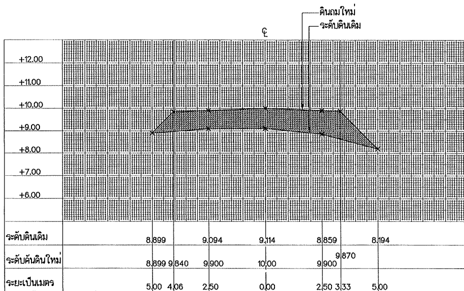
รูปตัด STA. 0+850
